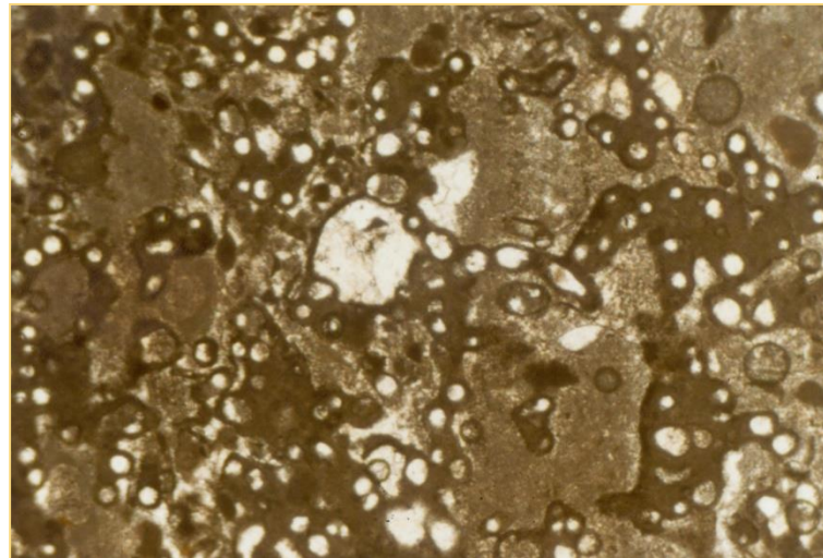
中华枝管藻横剖面
