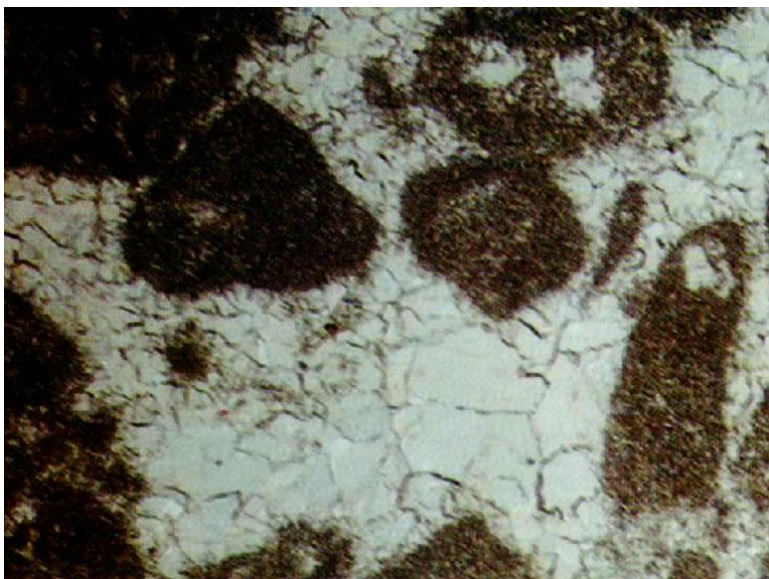
亮晶砂屑石灰岩
