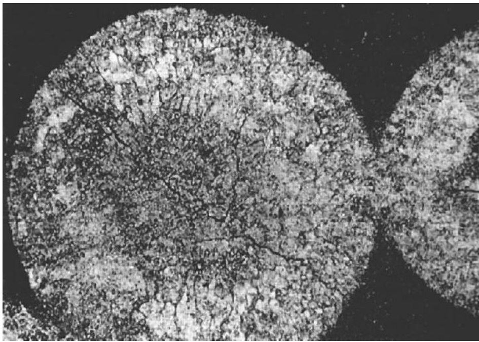
泥晶鲕粒灰岩，结构退变
